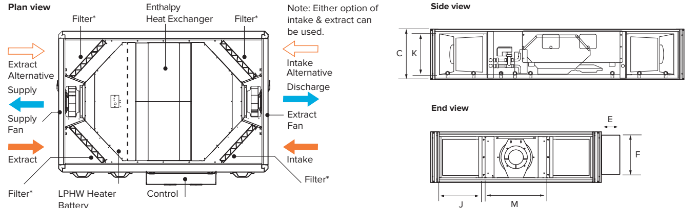
FAN CONFIGURATION
