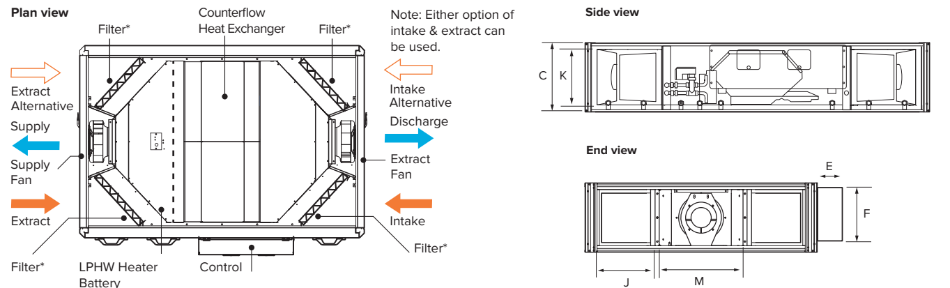
FAN CONFIGURATION
